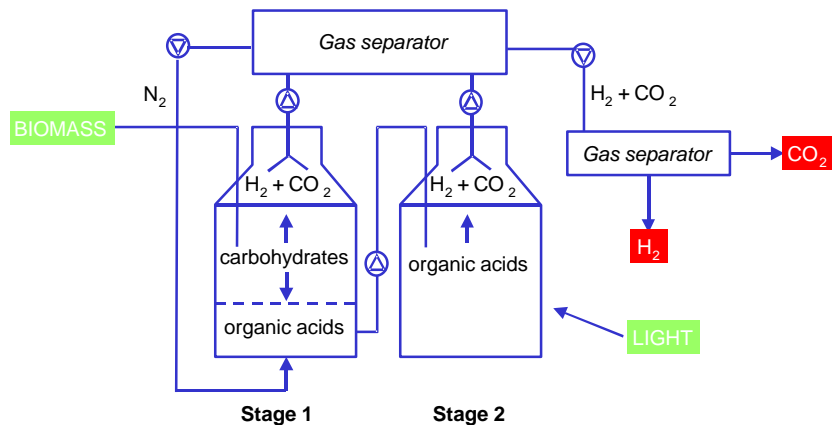
Productie van H 2 uit biomassa in een 2 stappen fermentatie.
